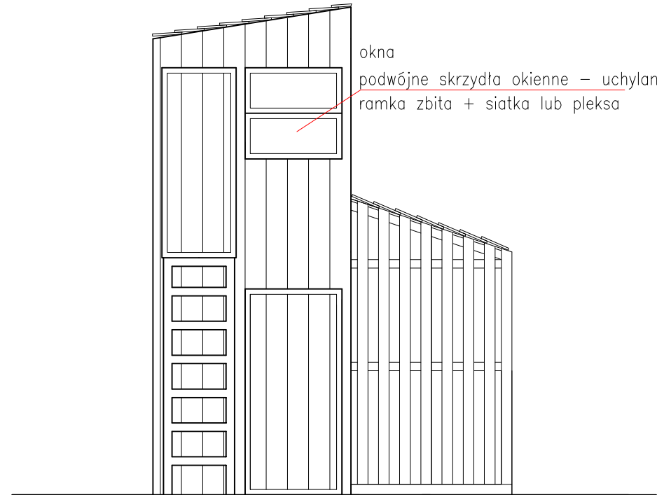
ELEWACJA WSCHODNIA
